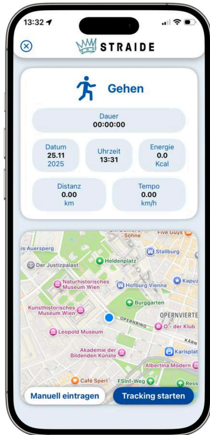
Tracking-Oberfläche
